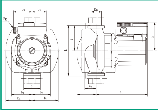
尺寸圖 A
