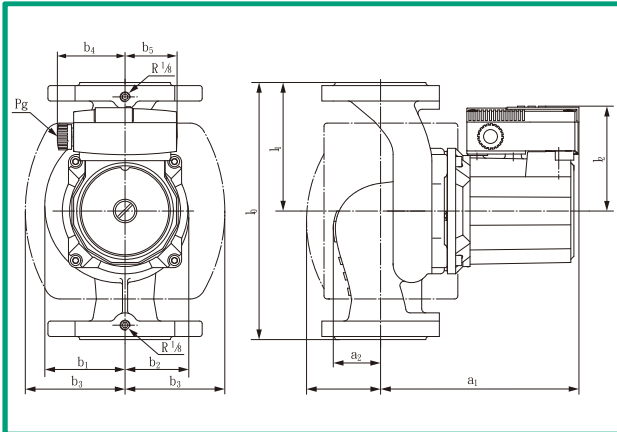
尺寸圖 C
