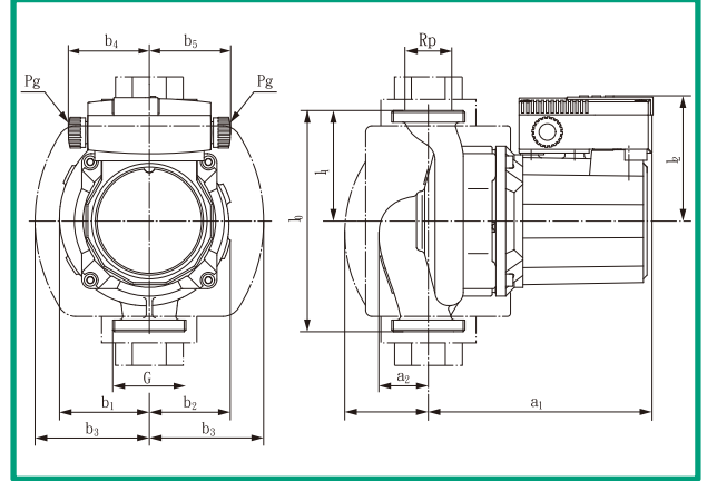
尺寸圖 B
