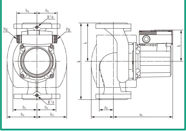
尺寸圖 D
