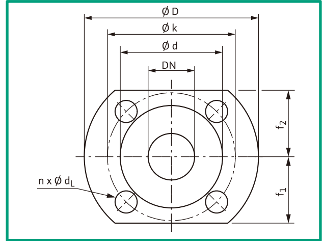
法蘭圖 G
