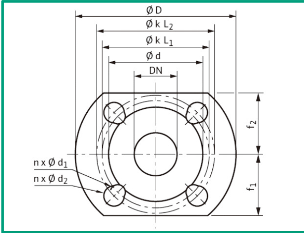
法蘭圖 F
