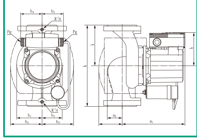
尺寸圖 E
